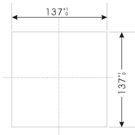
图 86 仪表开孔尺寸
