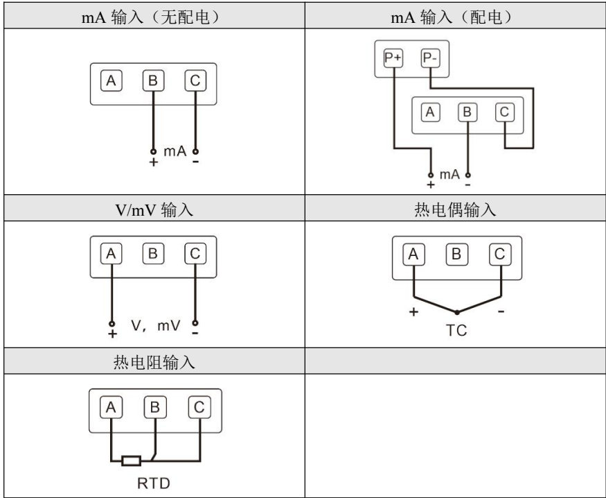
图 2-5 信号线连接示意图
