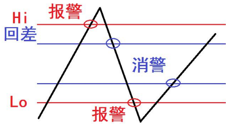
图 4-1 高低报警及回差图例
