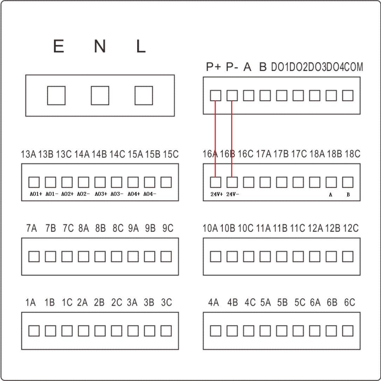
图 2-4 增强型端子视图
