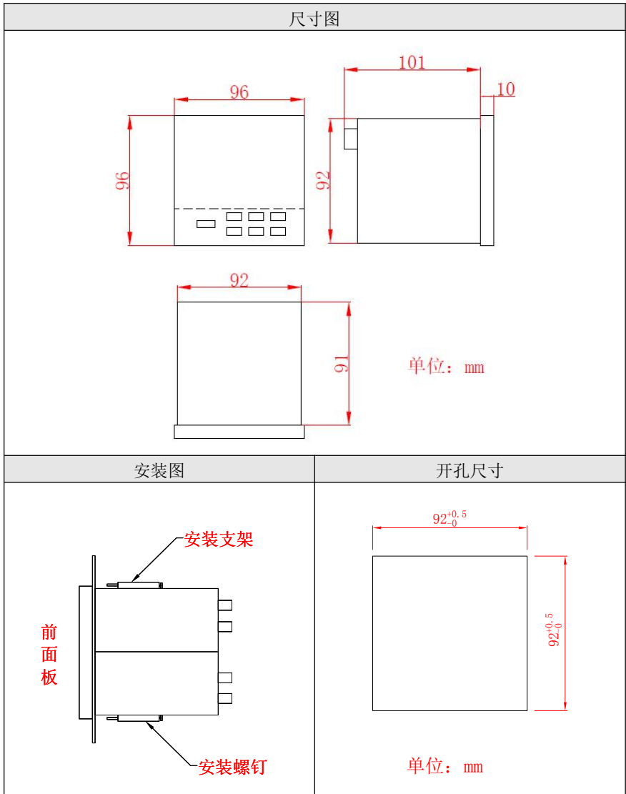
图 2-2 产品尺寸及安装图
