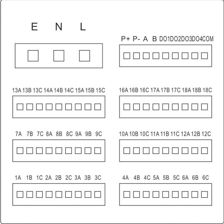
图 2-3 基础型端子视图
