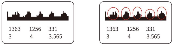
图 50 变频器干扰的回波图形
