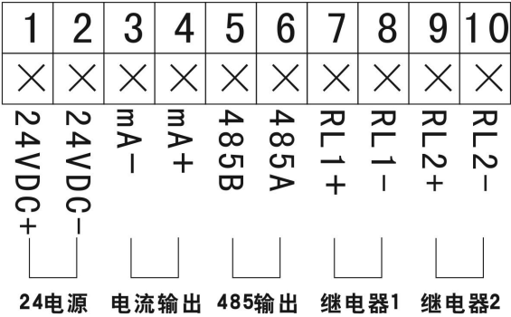
图 39 四线制 24VDC 供电接线图
