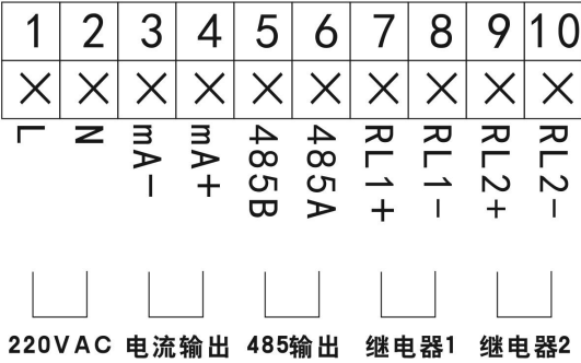
图 40 四线制 220VAC 电气连接图
