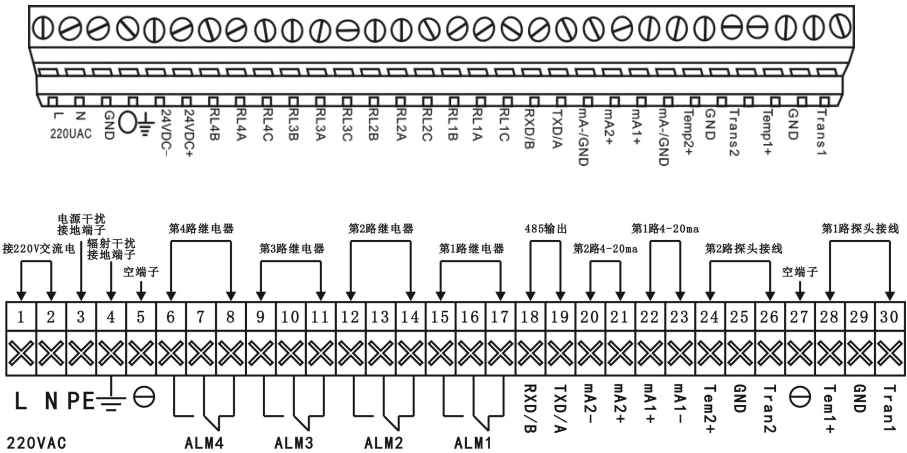
图 37 电气连接图和接线端子示意图
