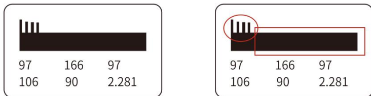
图 54 探头缩在接管内的回波
