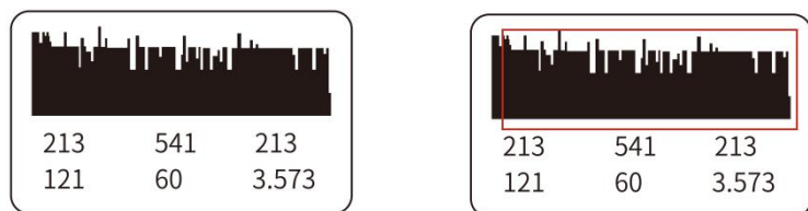
图 53 强烈干扰的回波图形
