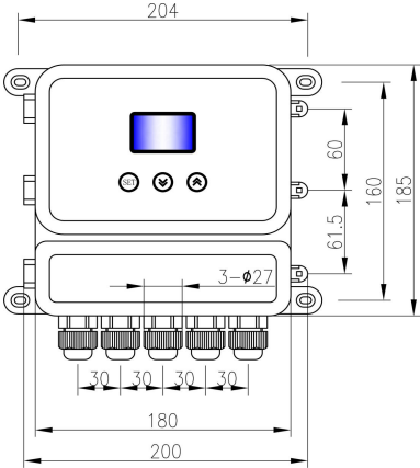
图 3 结构图
