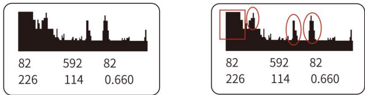
图 46 进入盲区后出现的回波图
