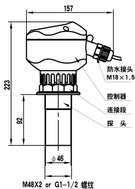
M48×2 或 G1-1/2 螺纹传感器 M60×2 或者 G2 螺纹传感器
