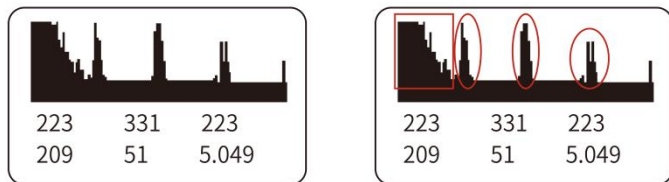
图 44 共振形成的回波信号
